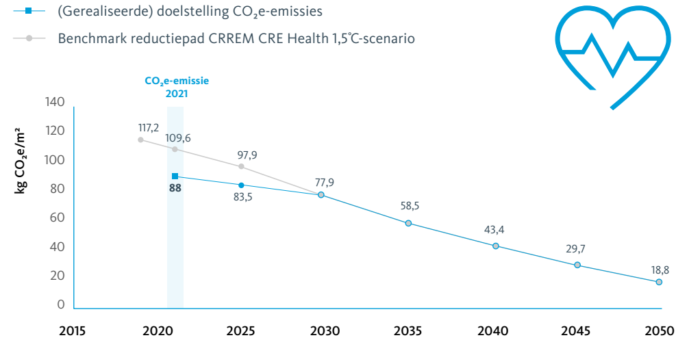
Figuur 10: Emissiereductiepad voor zorg (in kg CO 2 e/m 2 )
