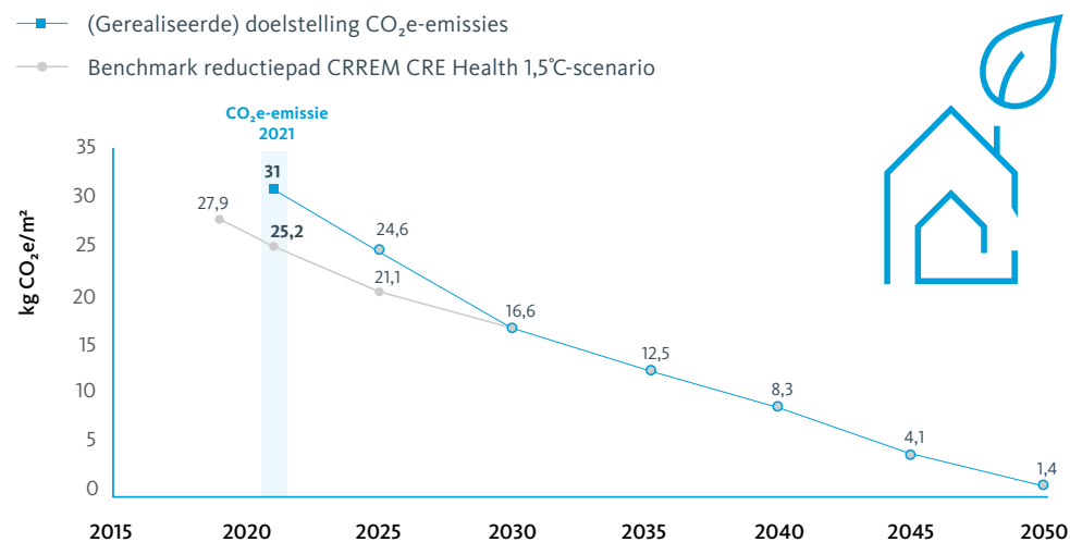
Figuur 8: Emissiereductiepad voor woningcorporaties (in kg CO 2 e/m 2 )
